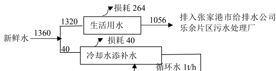
图 2-1 本项目水量平衡图（单位：t/a）
