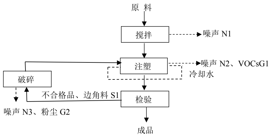
图 2-2 塑料制品生产工艺流程图
