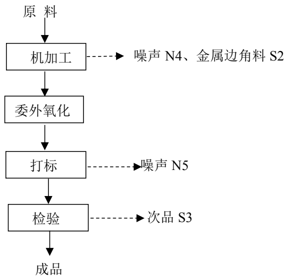
图 2-2 金属制品生产工艺流程图
