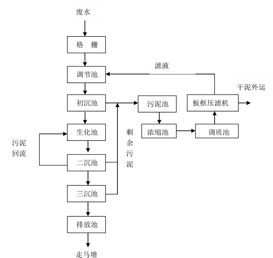
清泉污水处理工艺流程图
